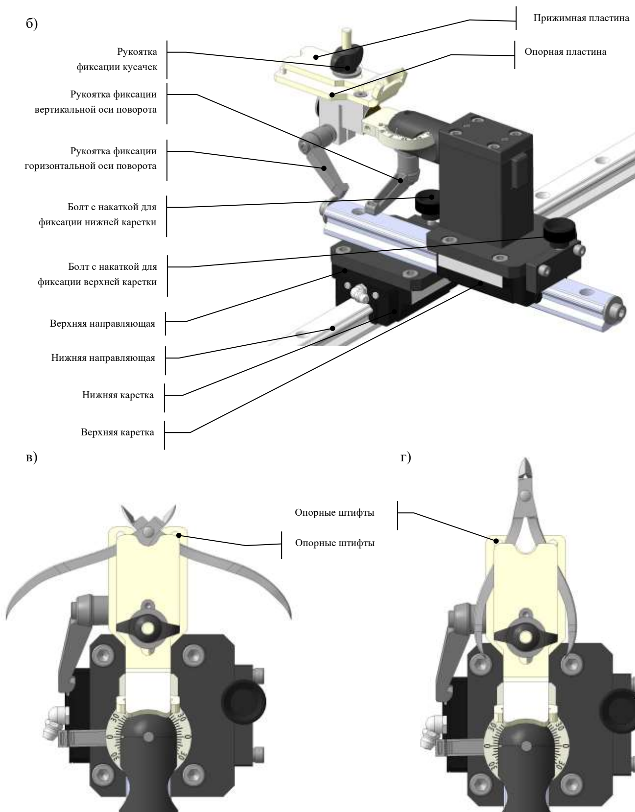
Рис.3 Станок ADEMS GMT-II
