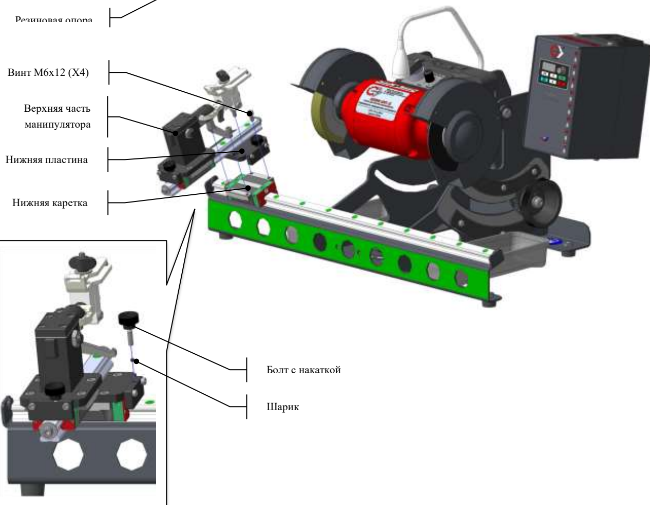
Рис.1 Сборка станка ADEMS GMT II
