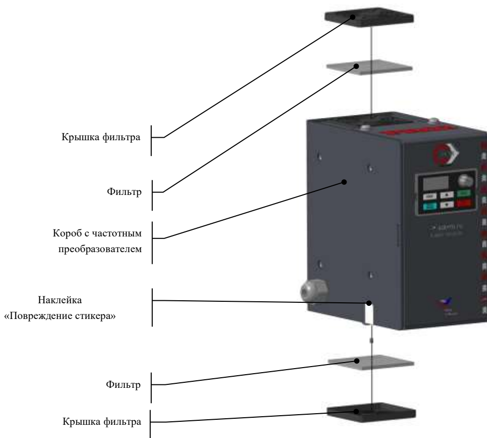
Рис. 10. Разборка и чистка фильтров
