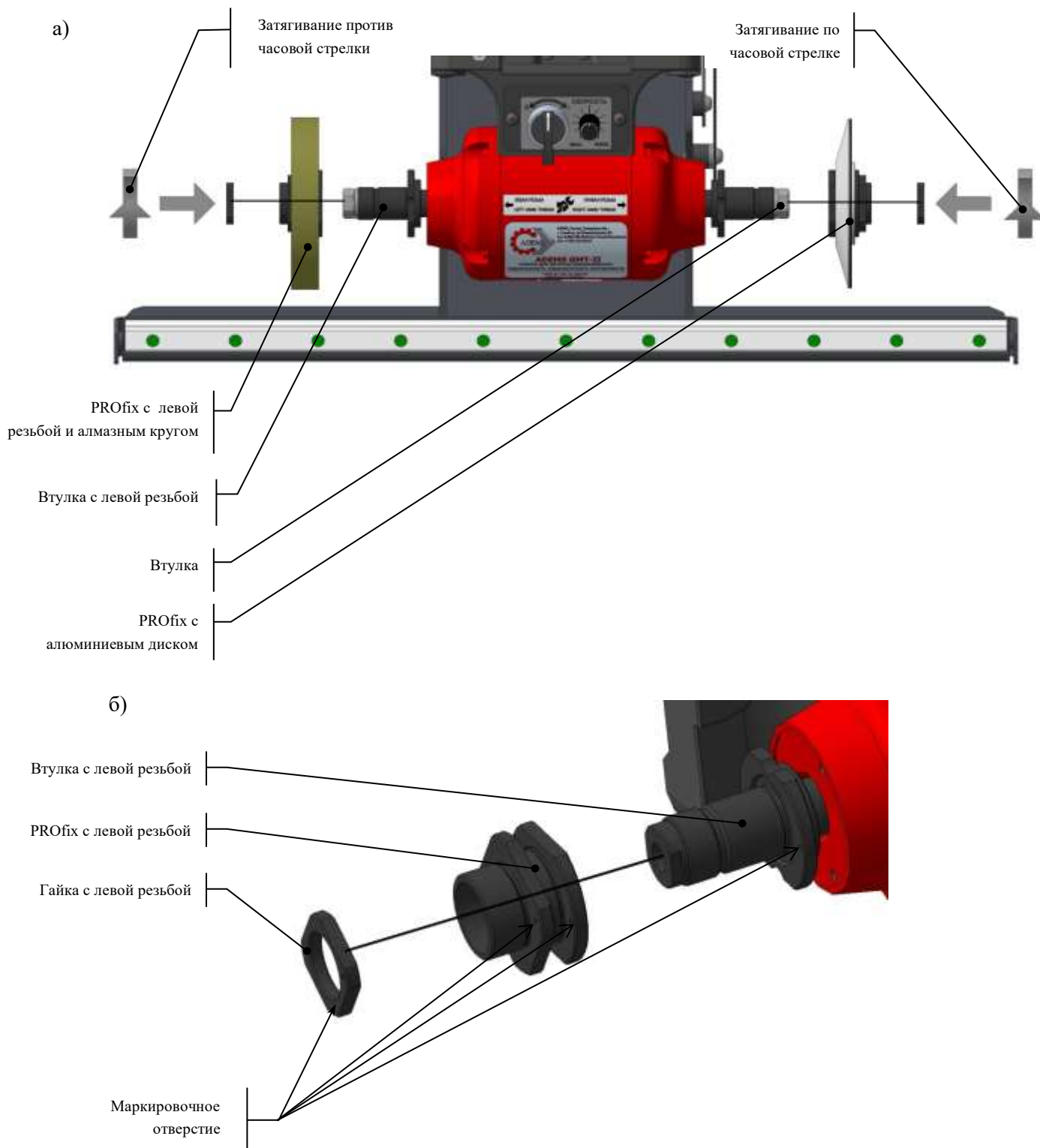
Рис.4 Положение PROfix на станке
